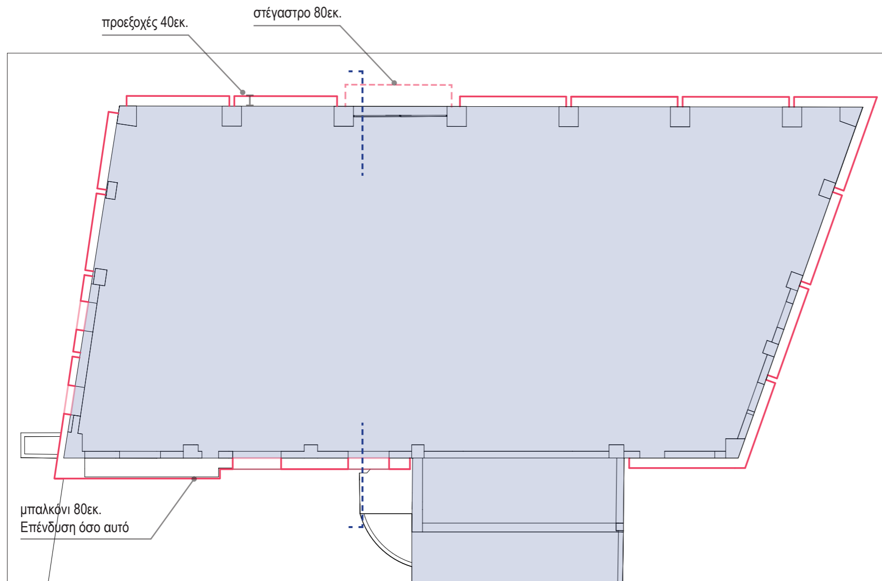
ΚΑΤΟΨΗ
