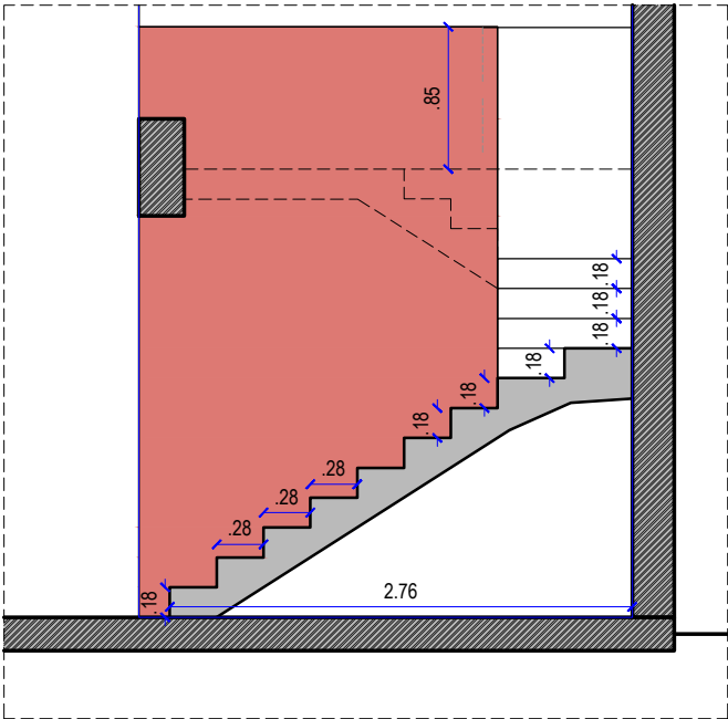
ΤΟΜΗ B-B'
