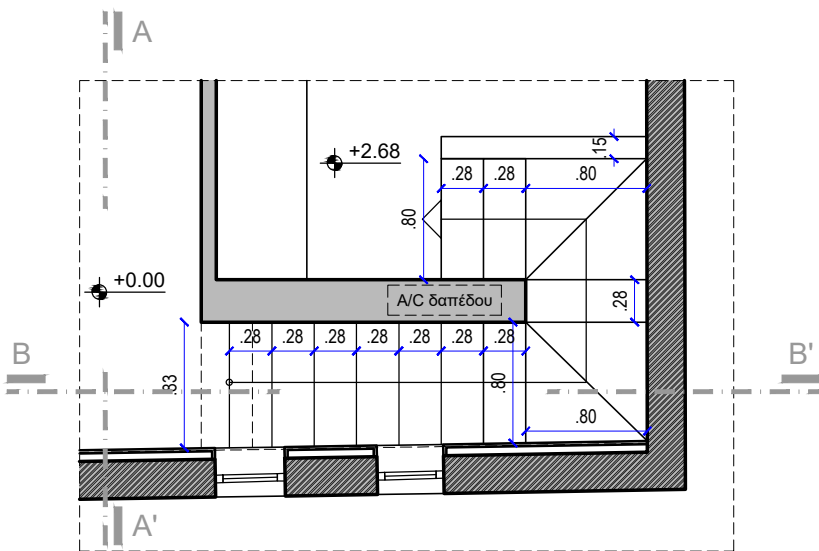
ΚΑΤΟΨΗ
