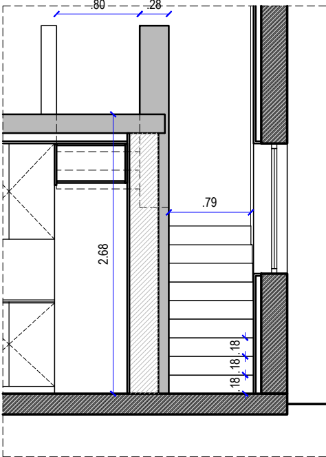
ΤΟΜΗ A-A'
